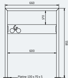
Version avec signalétique sur platines - Réf. 294018
