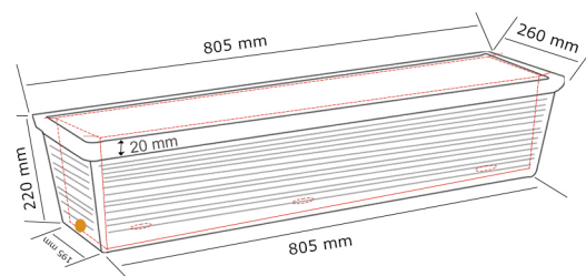
P-BAL-800-A (Contre bac inclus) Poids : 5 kg Volume : 25 L
