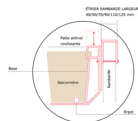
Fixation pour version Suspendue
