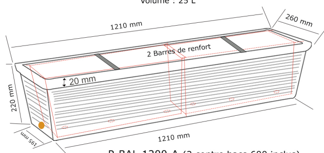
P-BAL-1200-A (2 contre bacs 600 inclus) Poids : 7.7 kg Volume : 44 L
