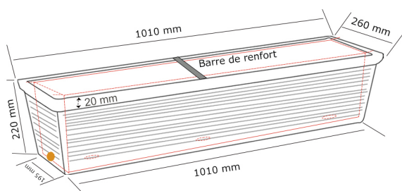
P-BAL-1000-A (Contre bac inclus) Poids : 6.25 kg Volume : 32 L
