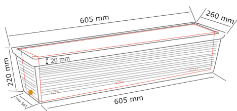
P-BAL-600-A (Contre bac inclus) Poids : 3.35 kg Volume : 22 L
