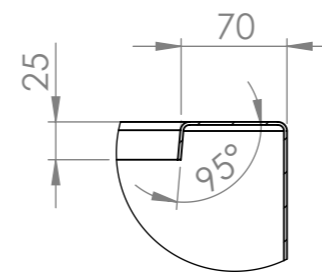
SECTION A-A SCALE 1 : 15
