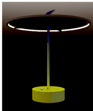
OPTION ECLAIRAGE LED alimentation autonome par panneau photovoltaïque et batterie ou raccordement au réseau électrique
